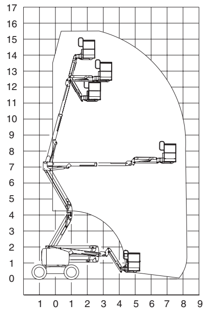
Cuadro de amplitud de movimientos de Z-45/25J
