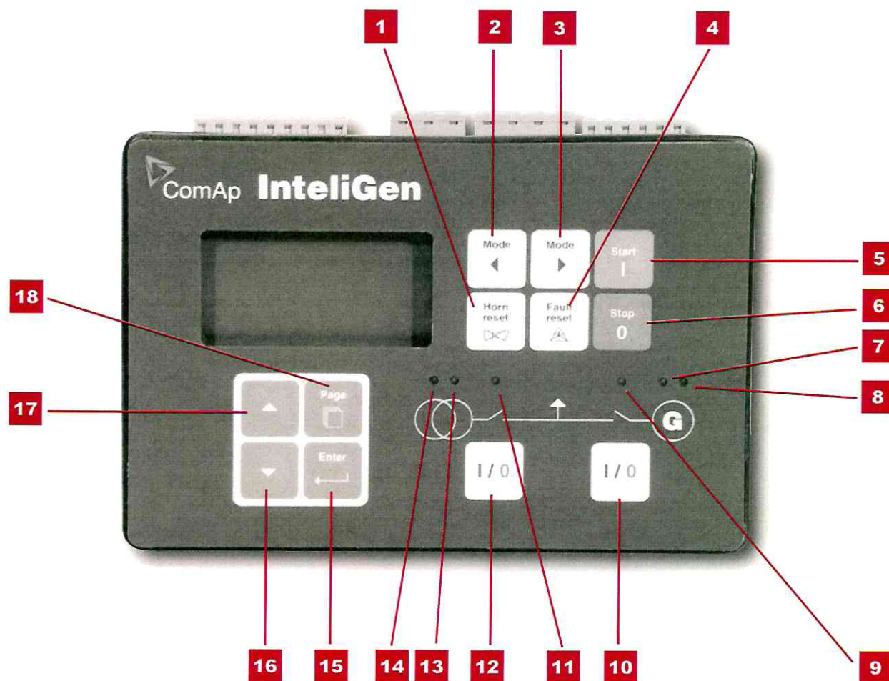
Imagen 14 - PLACA DE CONTROL INTELIGEN
