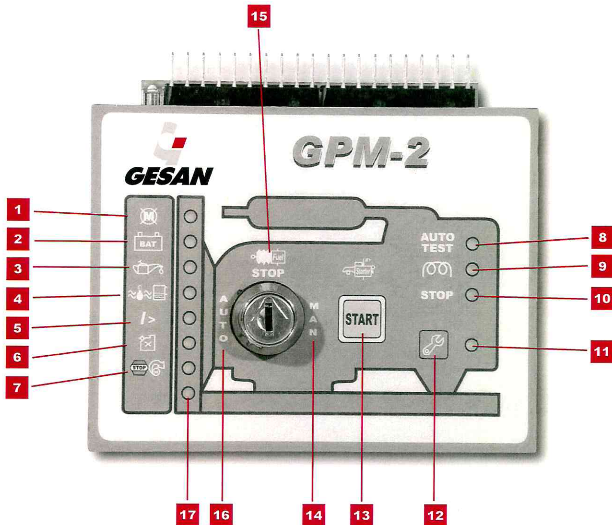
Imagen 10 - PLACA DE CONTROL GPM-2
