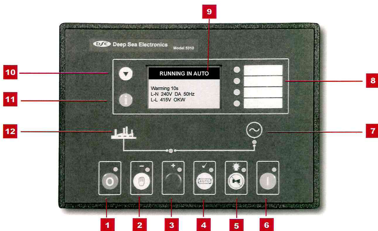
Imagen 13 - PLACA DE CONTROL DEEP SEA 5310
