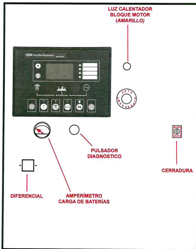
Imagen 6 - CUADRO DE CONTROL DE PLACA DE CONTROL DEEPSA
