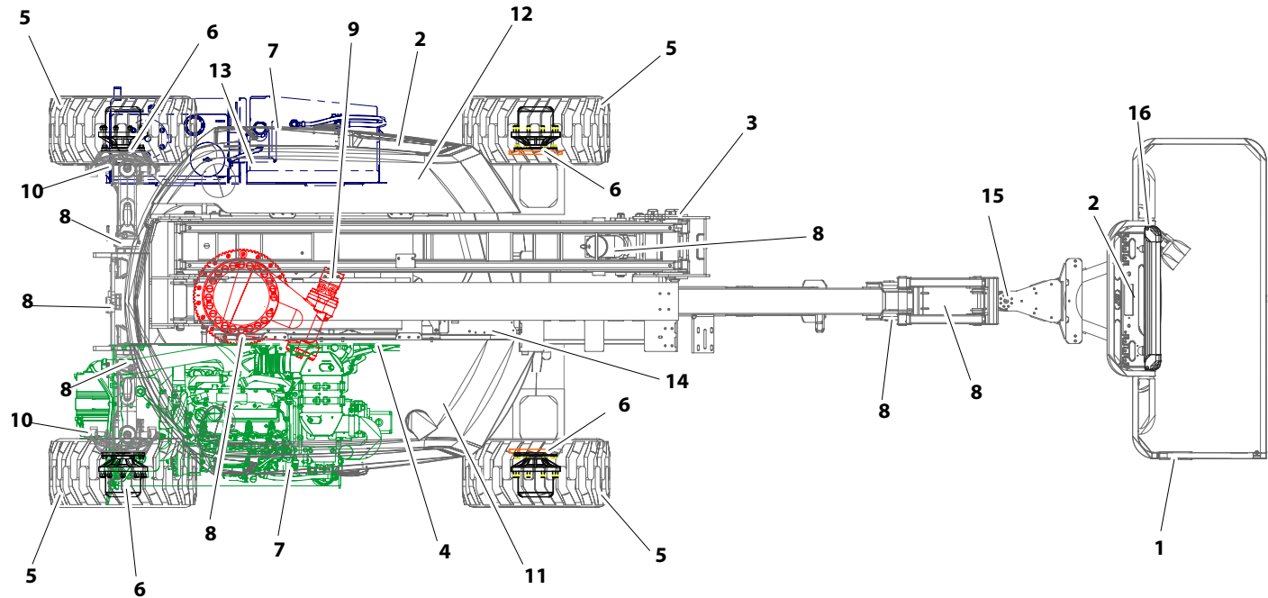
Figura 2-2. Inspección visual diaria: hoja 1 de 3
