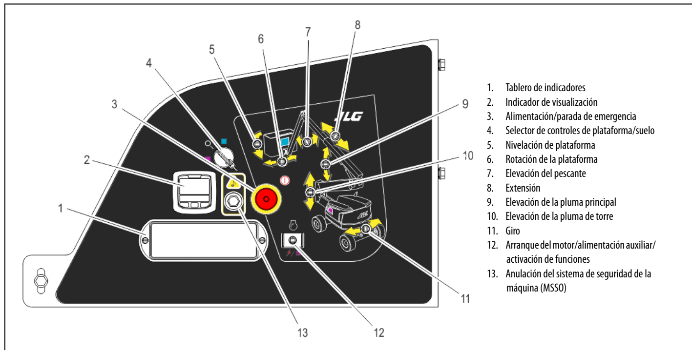
Figura 3-2. Consola de controles de suelo con MSSO (CE solo)
