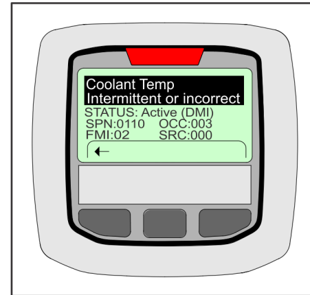
Figura 3-6. Pantalla de diagnóstico del motor
