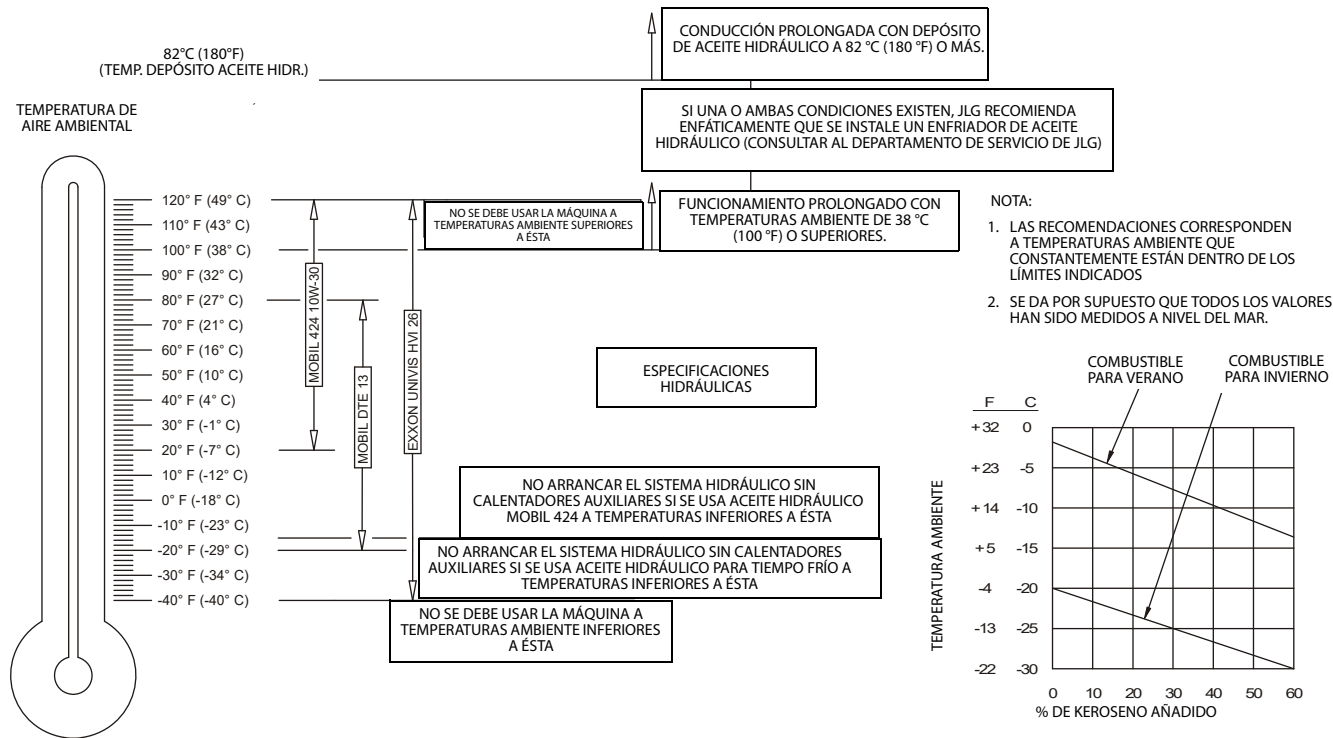
Figura 7-2. Especificaciones de temperatura de funcionamiento del motor – Deutz 2,3 I – Hoja 2 de 2
