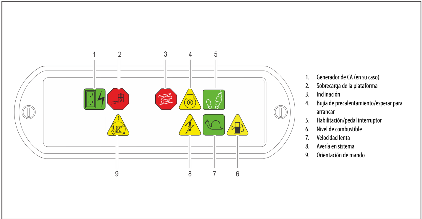
Figura 3-9. Tablero de indicadores en controles de plataforma
