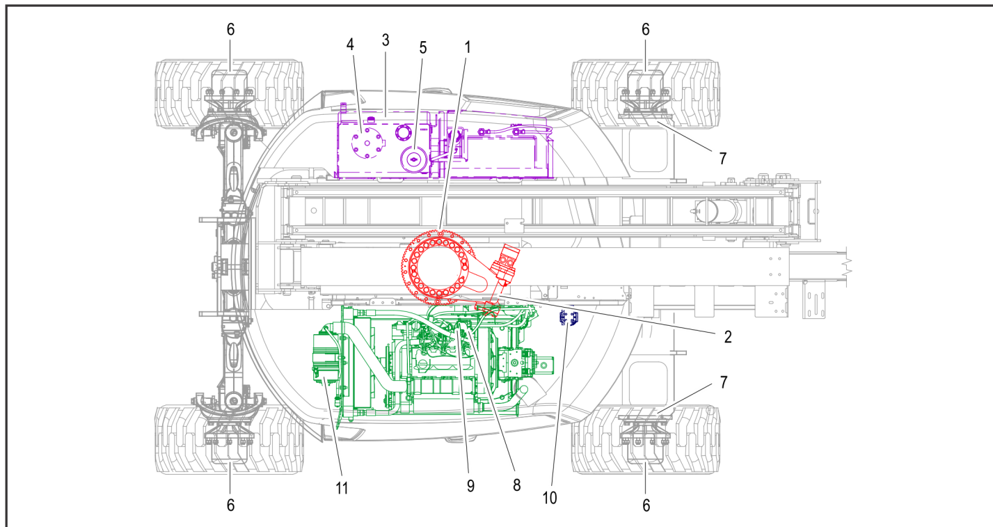
Figura 7-3. Diagrama de mantenimiento y lubricación por parte del operador
